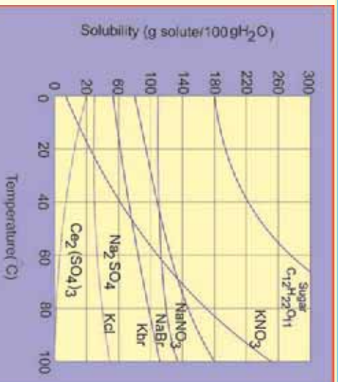
1-7 شکل په 100\text{g} اوبو کې د مالګې د حل کېدلو گراف
